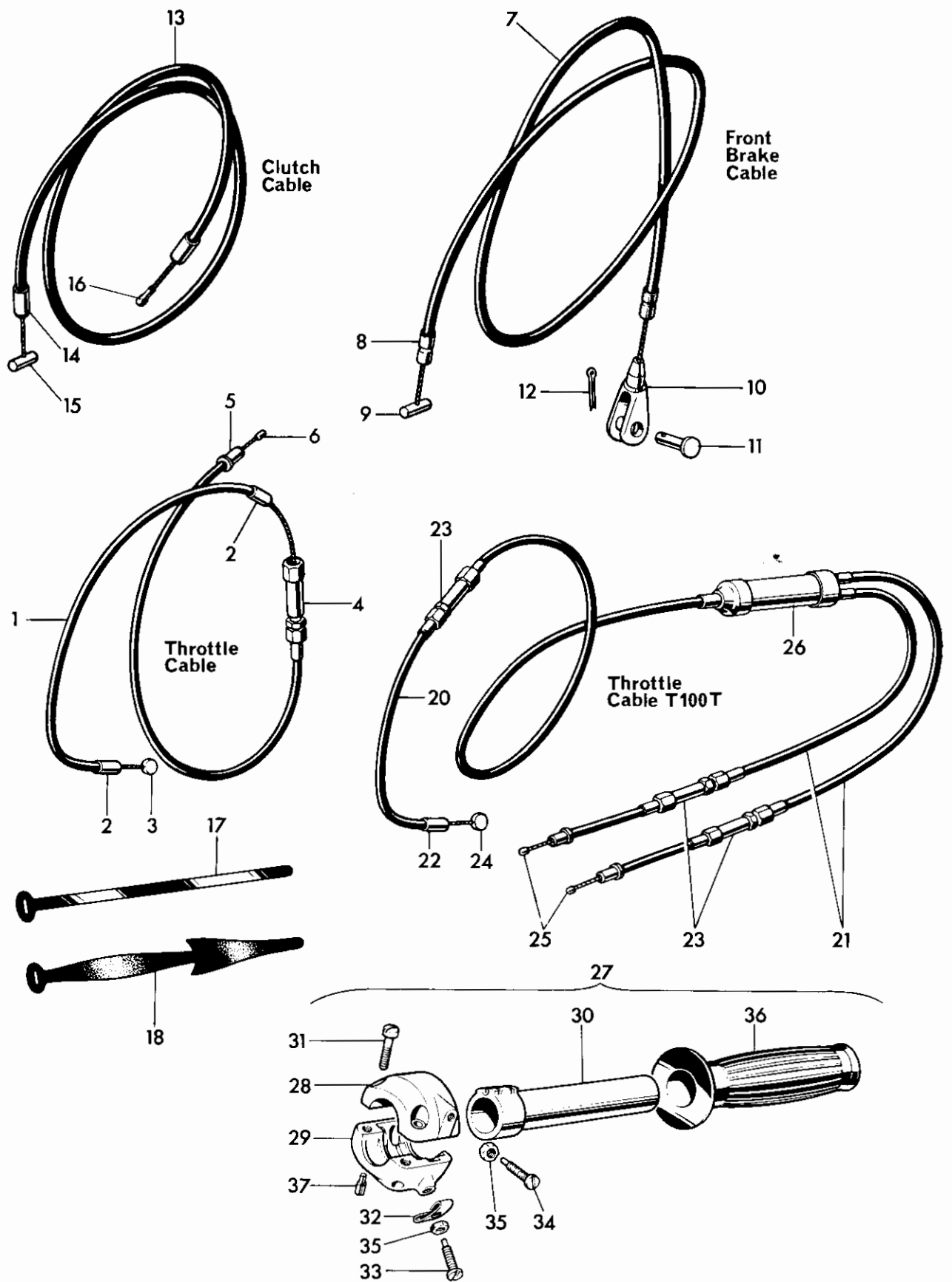
Fig. 28. CONTROL CABLES
